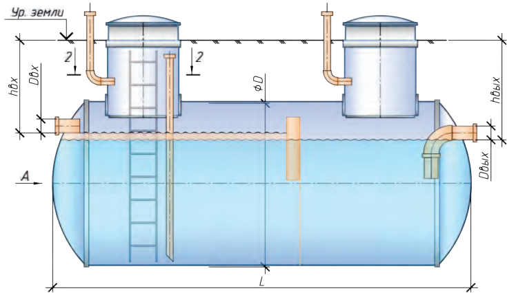
Горизонтальное исполнение
